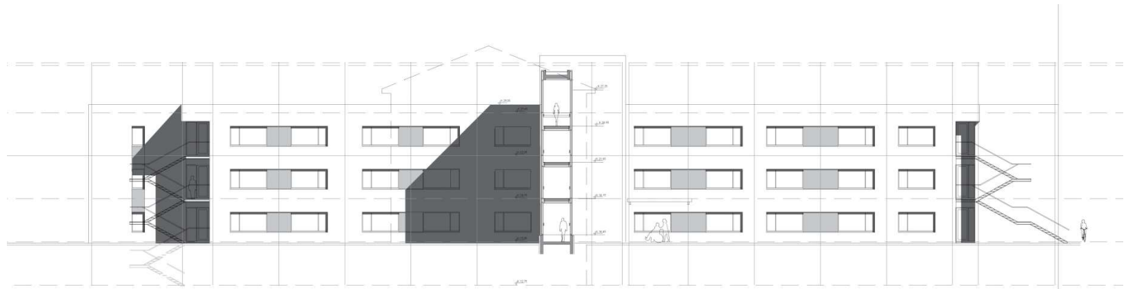
SNEIÐING D-D 1:100
